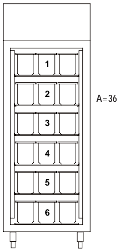
Bacinelle } H=180 Containers
