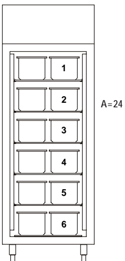
Bacinelle } H=180 Containers
