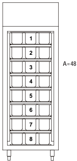
Bacinelle } H=150 Containers
